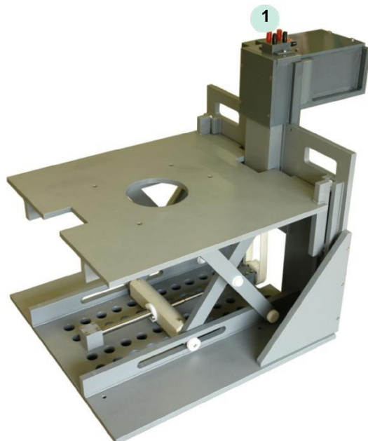
升降台前视图。
